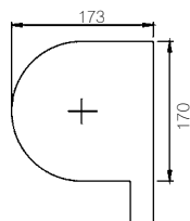
165er-Kasten
